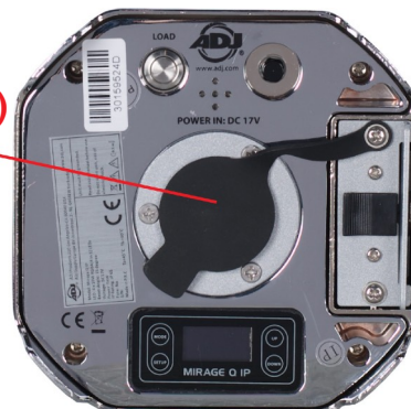
CAPUCHON DU PORT DE CHARGE (EN PLACE)
