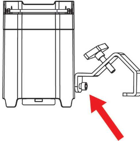
POINT DE FIXATION DE LA PINCE DE MONTAGE
